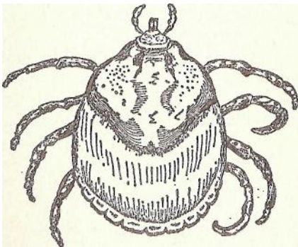
Fig. 1. La tique
